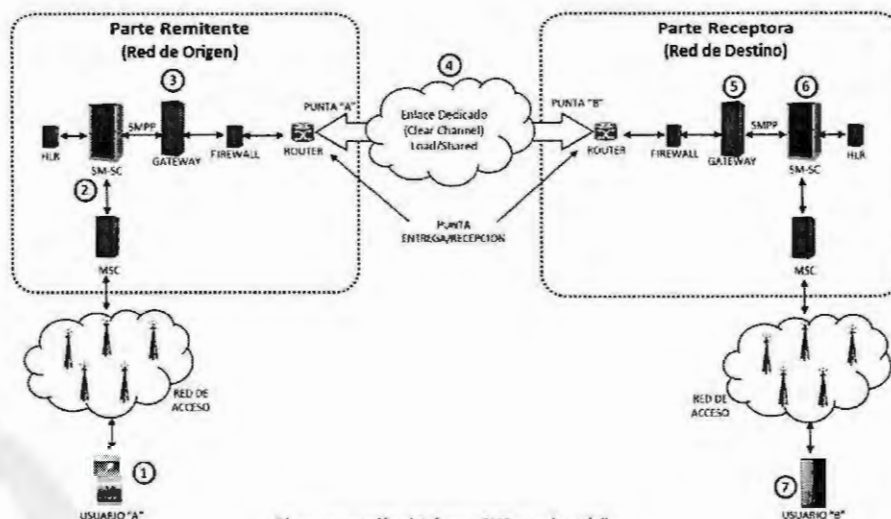
Diagrama conexión plataformas SMS en redes móviles
